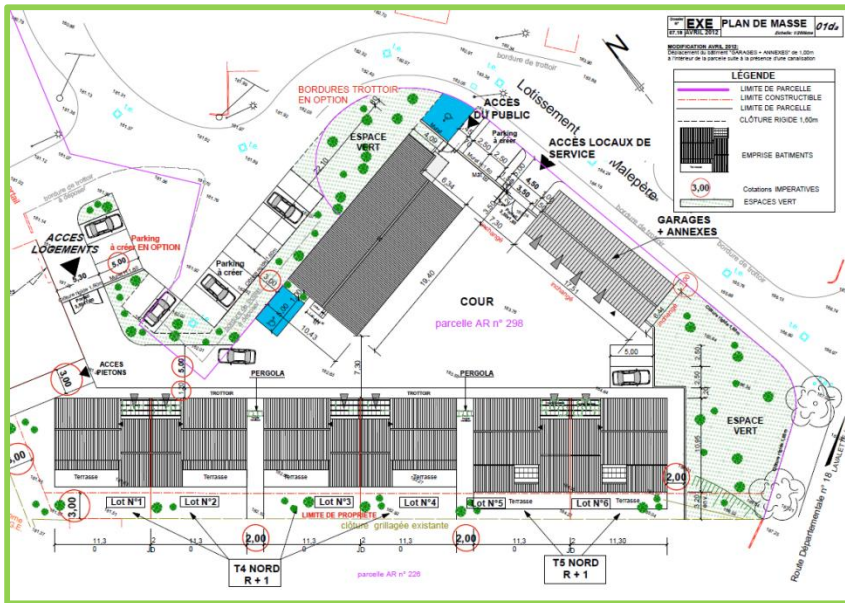
Plan de masse extension
