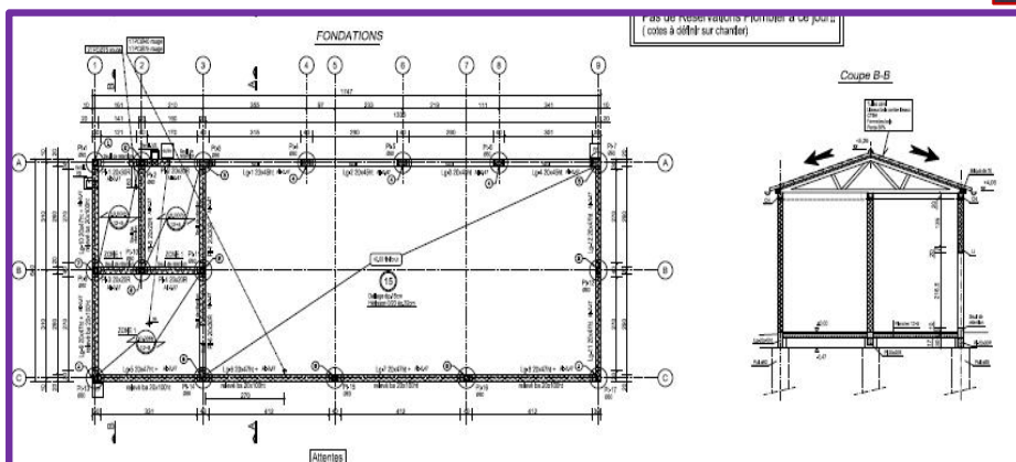
Extrait plan « fondations – RDC – coupes locaux techniques »
